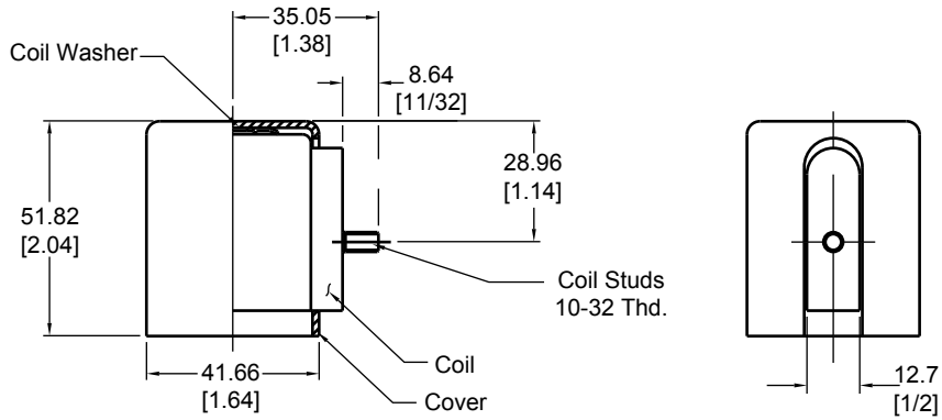
Single Stud
