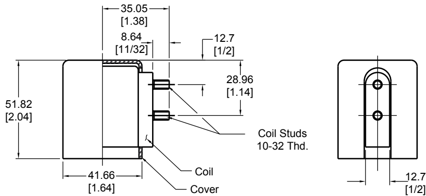
Double Stud
